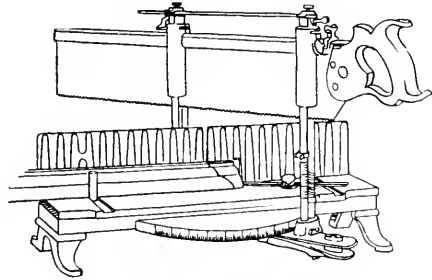
FIG. 214. MITER BOX.
